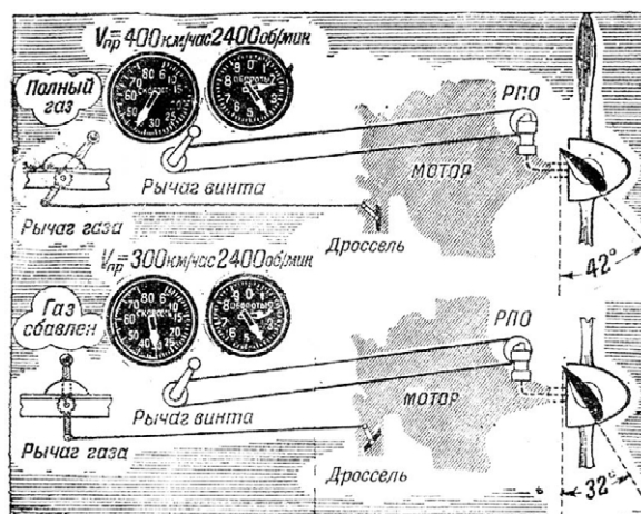
Рис. 16. Изменение шага автоматического винта, вызванное дросселированием мотора.
