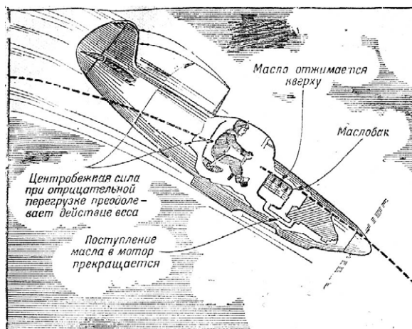
Рис. 24. Нарушение работы системы маслопитания при вводе самолета в пикирование с отрицательной перегрузкой.
