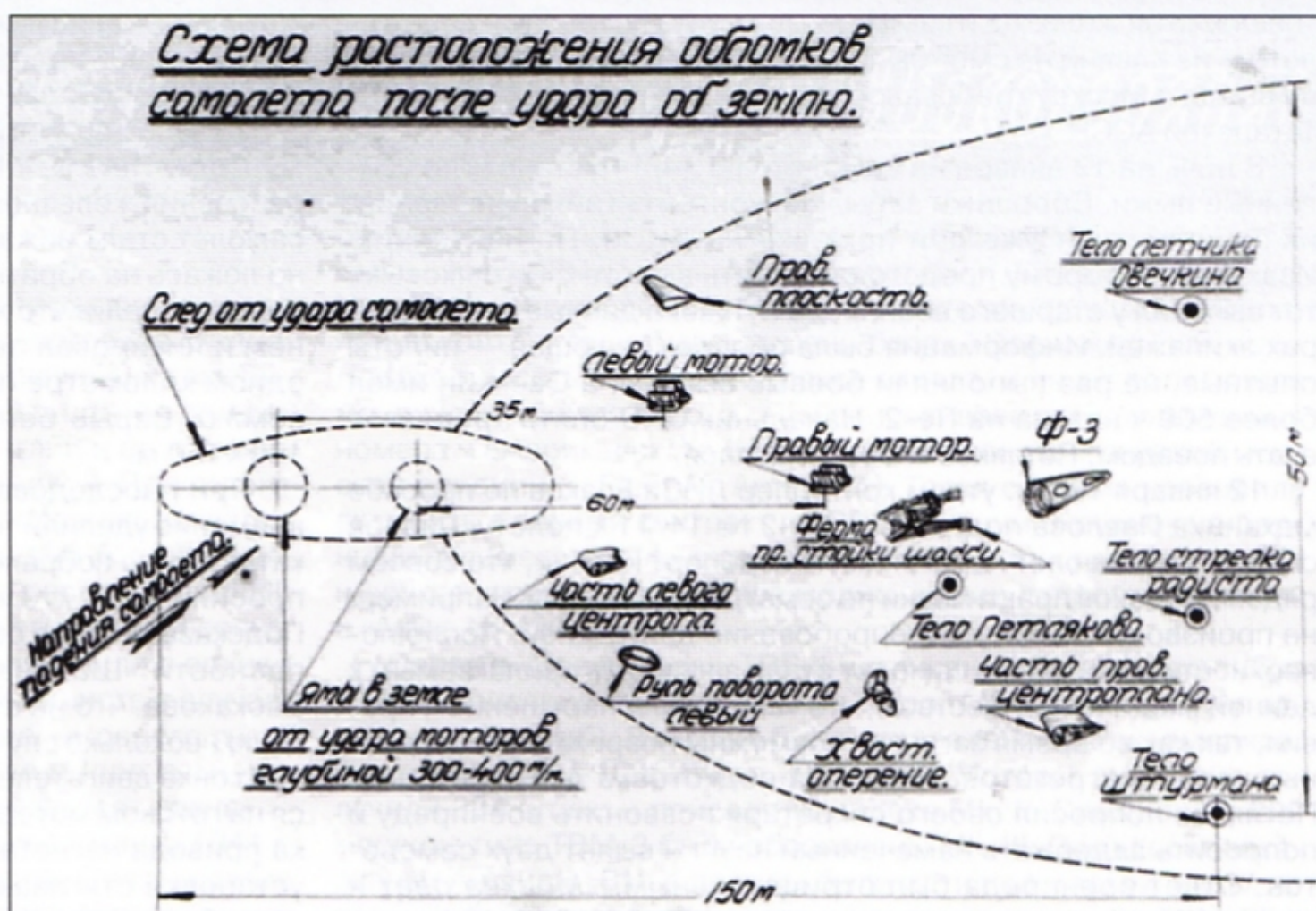
Схемы катастрофы Пе-2 № 14/11 и расположения его обломков
