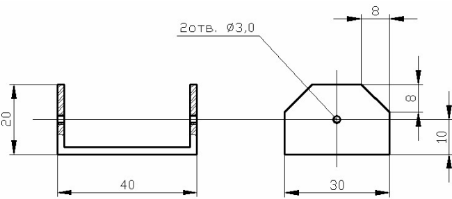
Рис. 5. Чертёж стойки стереоскопа (Б)
